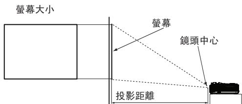
投影距離 vs 投影尺寸 (4:3)
